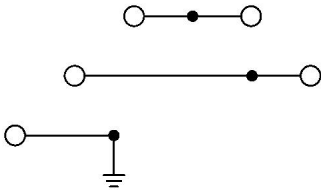
电路图
