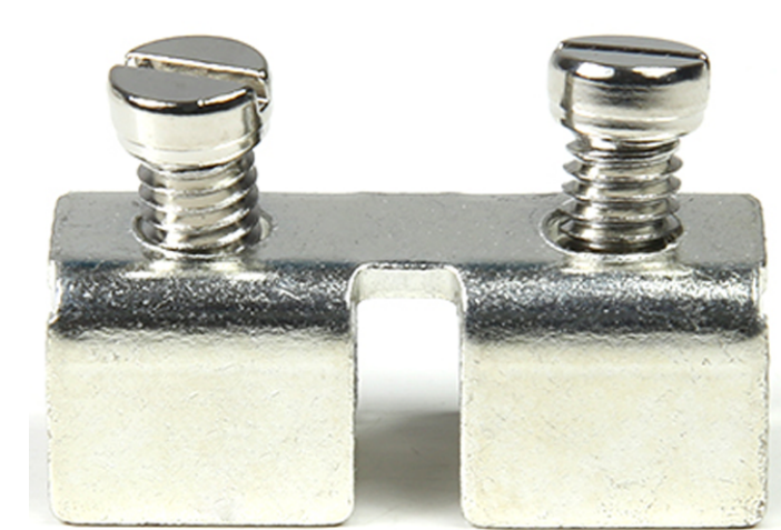
中心式联接件，中心距：20mm，位数：2，颜色：银色
