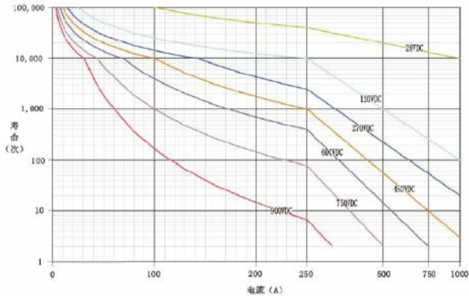
UQR100 负载切换寿命曲线图
