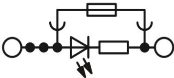
电路图
